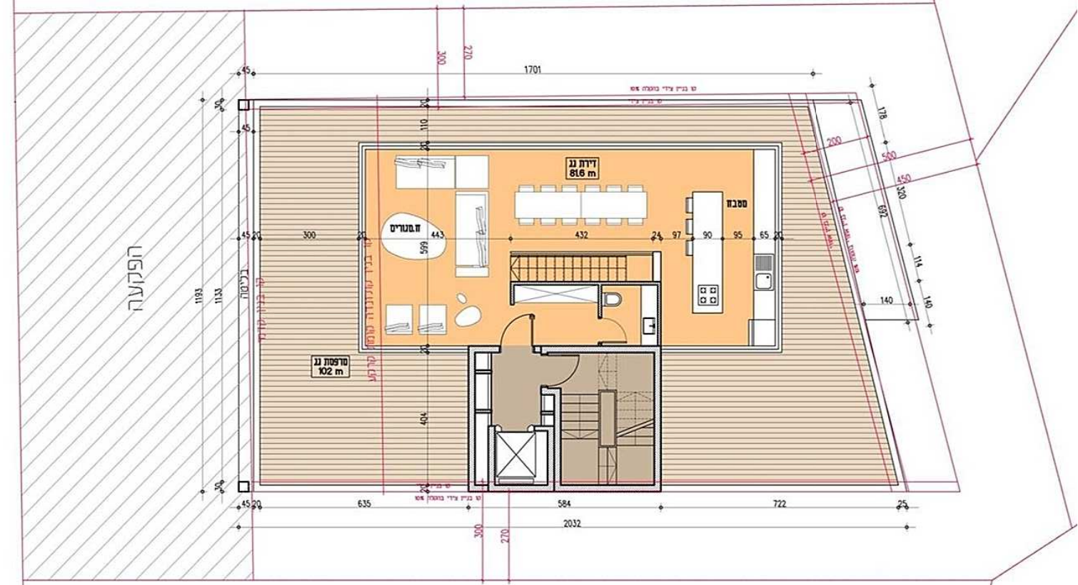
קומה 5 קנ"מ 1:100
